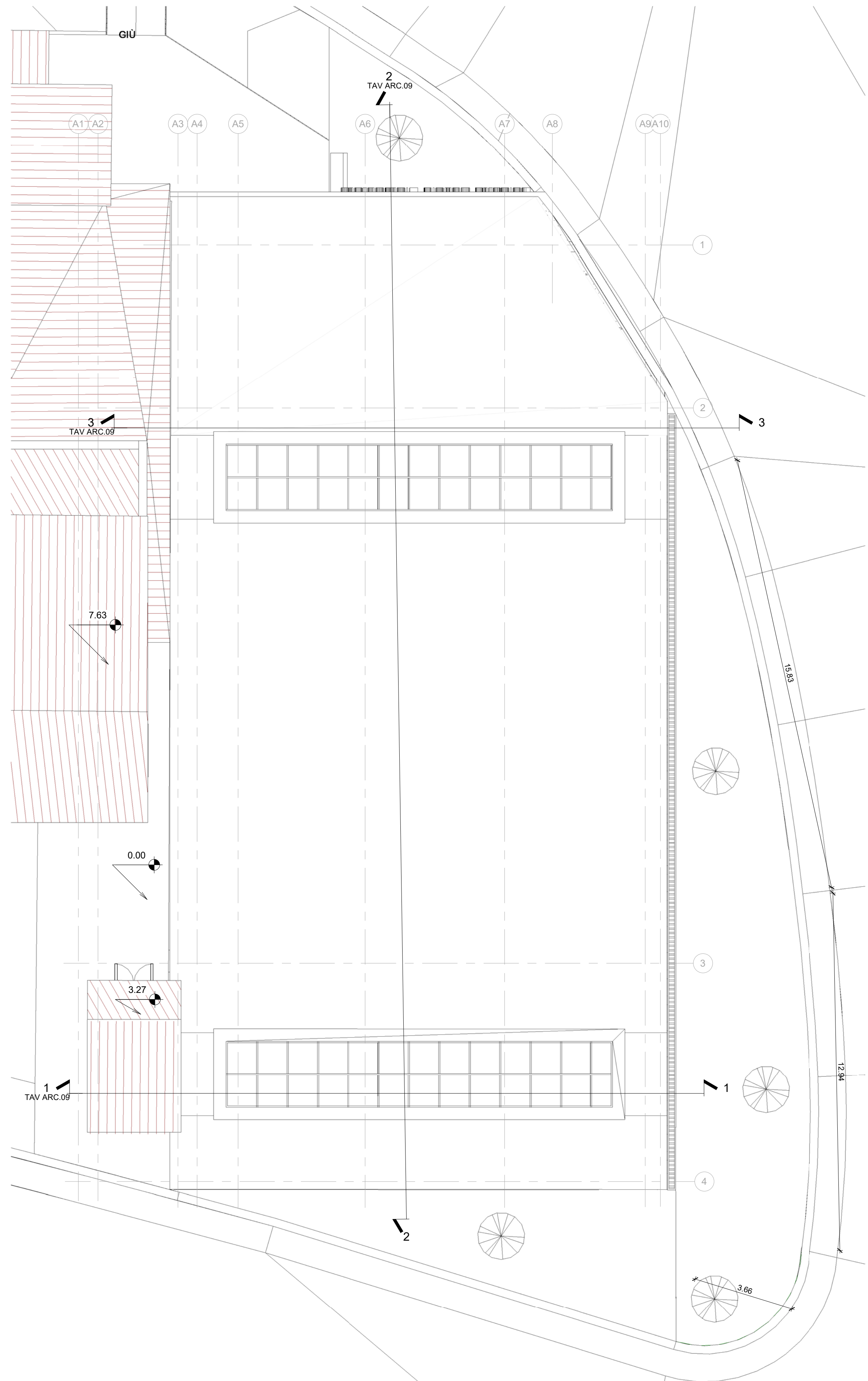
PIANTA LIVELLO COPERTURA Sc. 1:100
