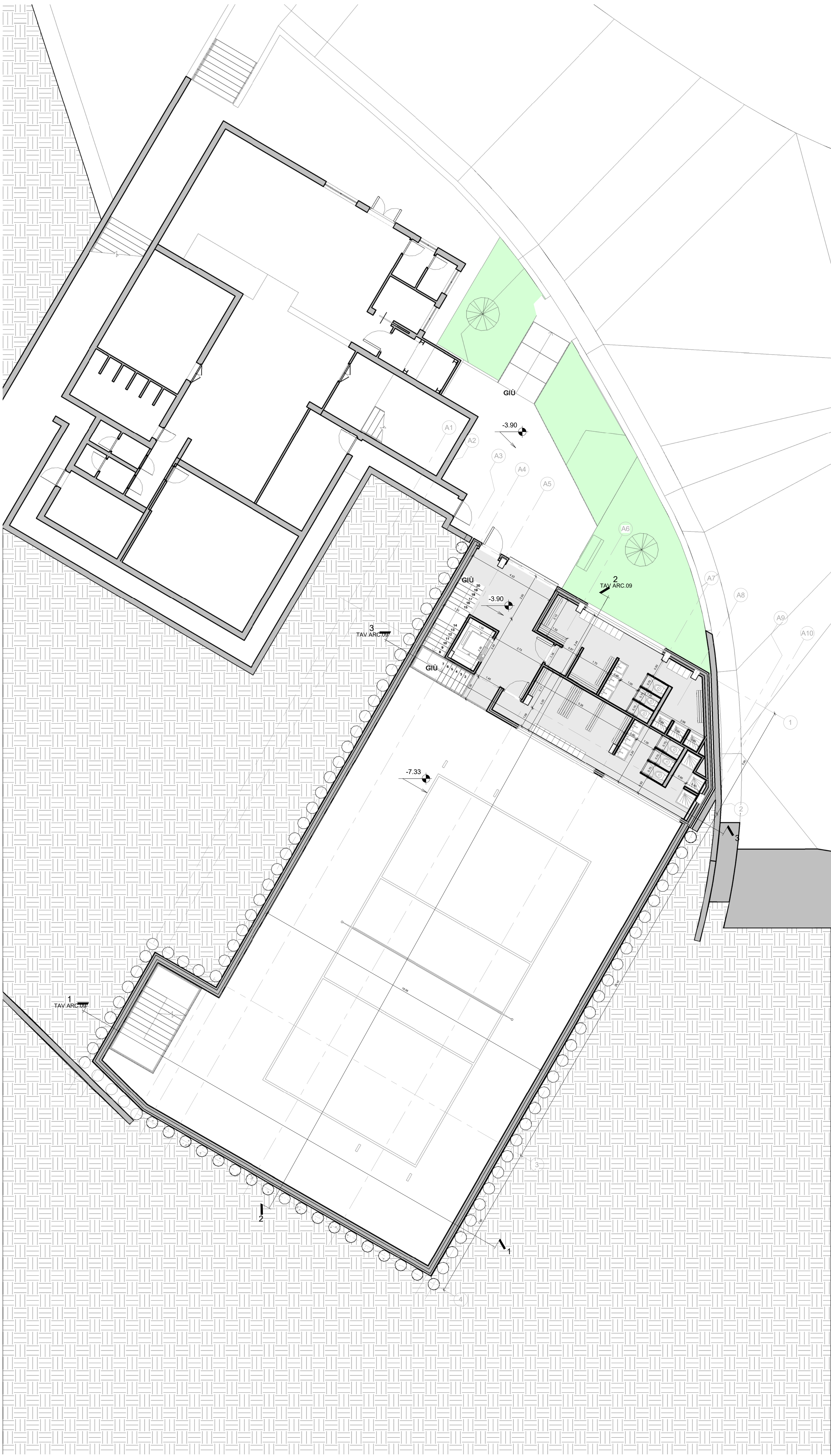
PIANTA LIVELLO -1 Sc. 1:100
