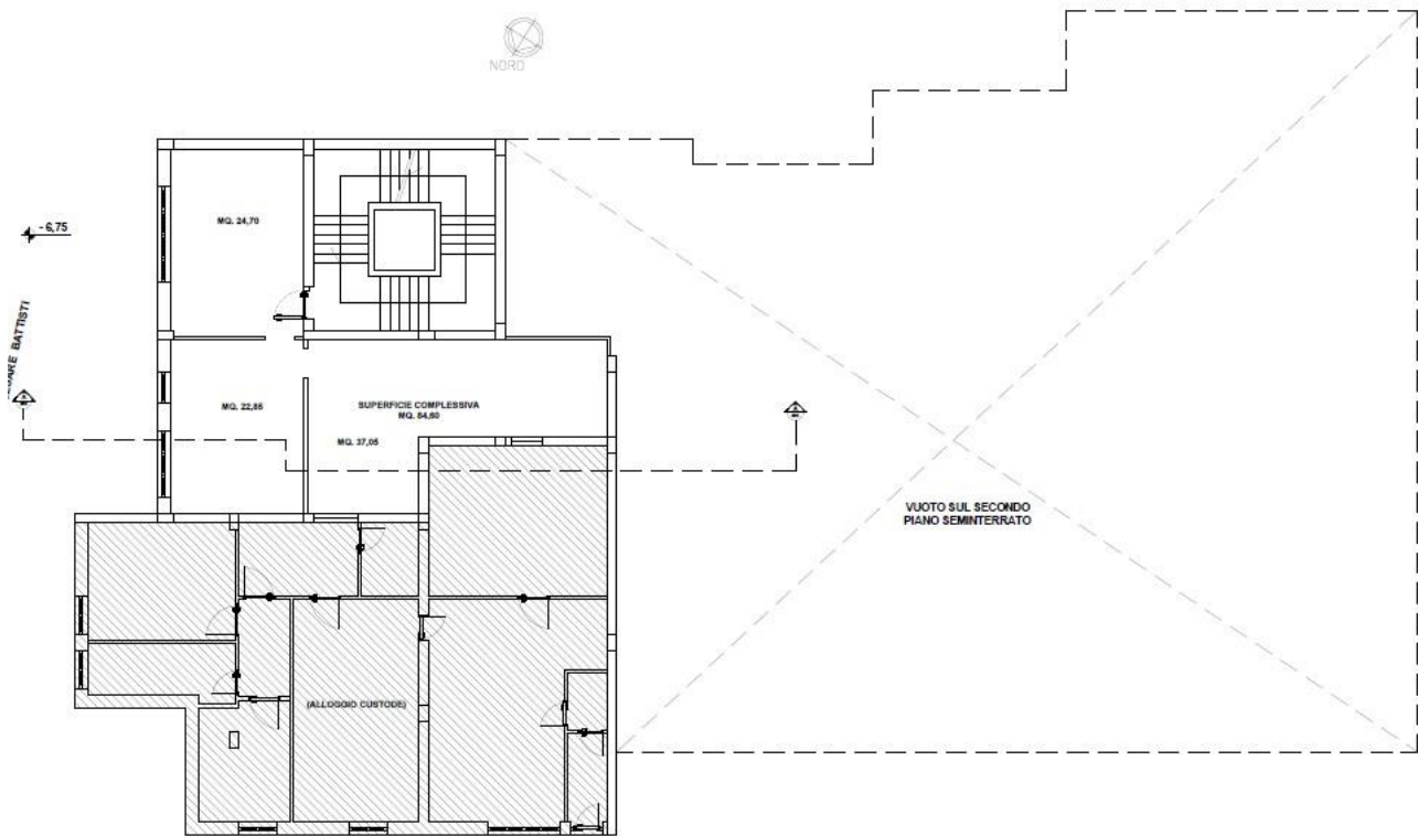
PIANTA PIANO PRIMO SEMINTERRATO rapp. 1:100
